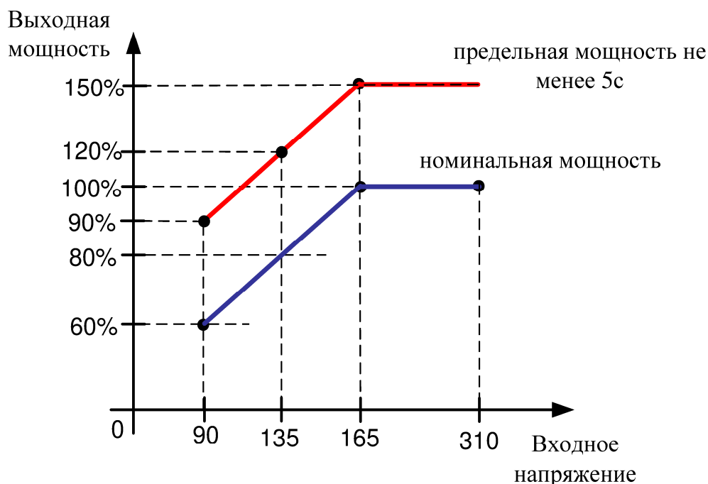
Рис. 5 – Зависимость выходной мощности от входного напряжения
